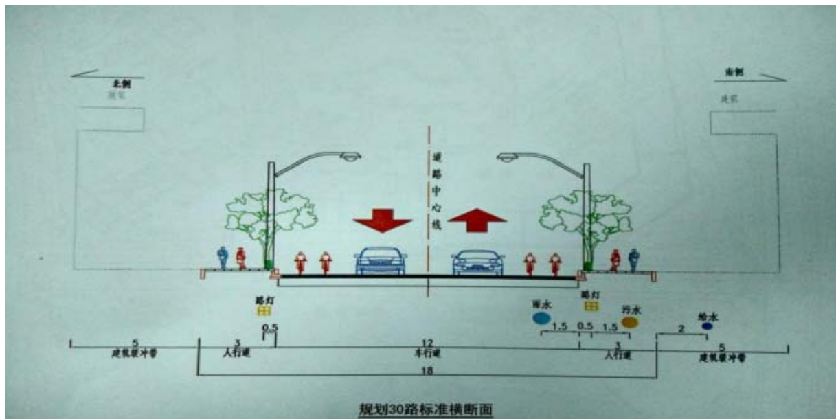
图 2 标准横断面
