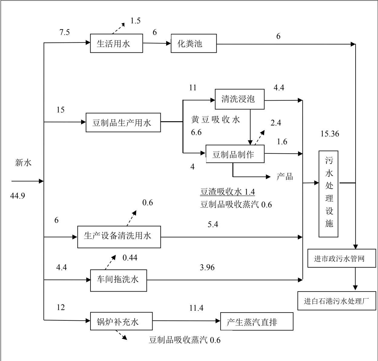
图 1 项目水平衡图 (单位: m³/d)
