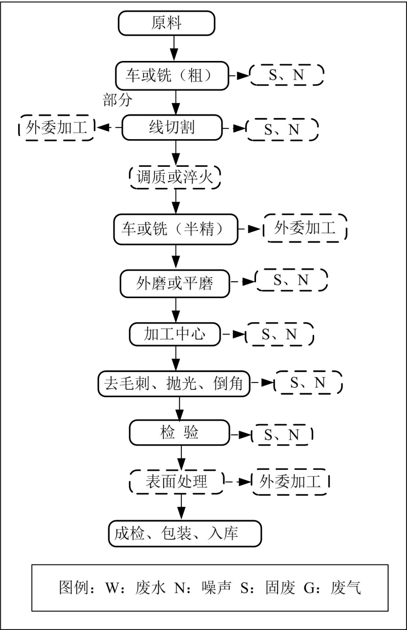
图 1 工艺流程及产污情况
