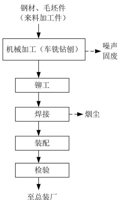
图 1 工艺流程及产污情况
