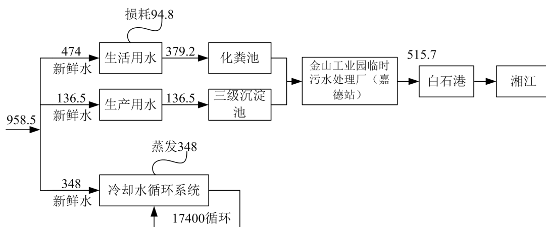
图 1 项目水平衡示意图（单位：m 3 /a）
