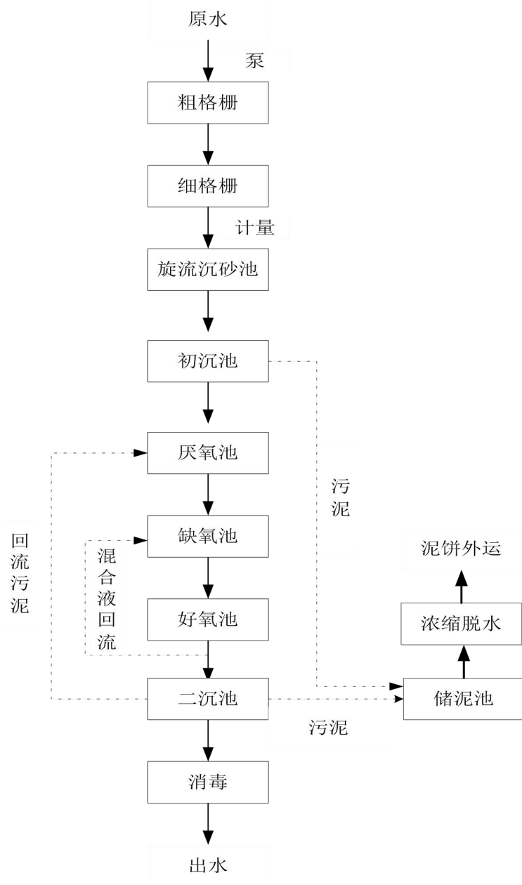
图 5 A 2 O 污水处理工艺
