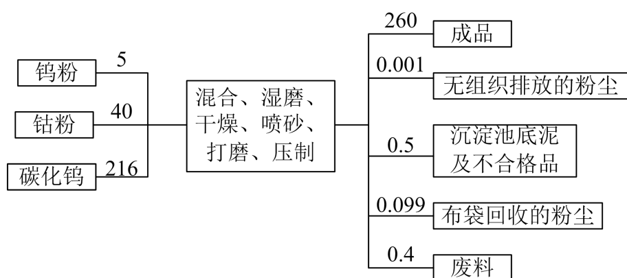
附图4 物料平衡图
