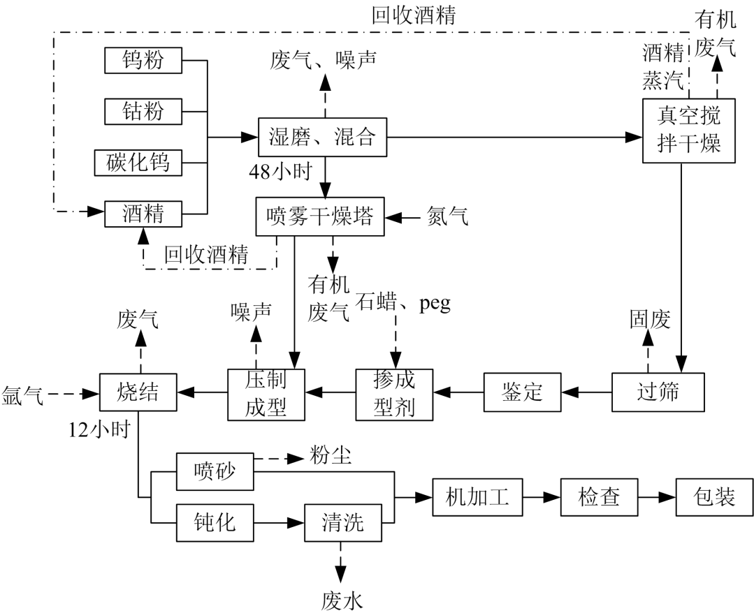
图2 工艺流程及产污情况
